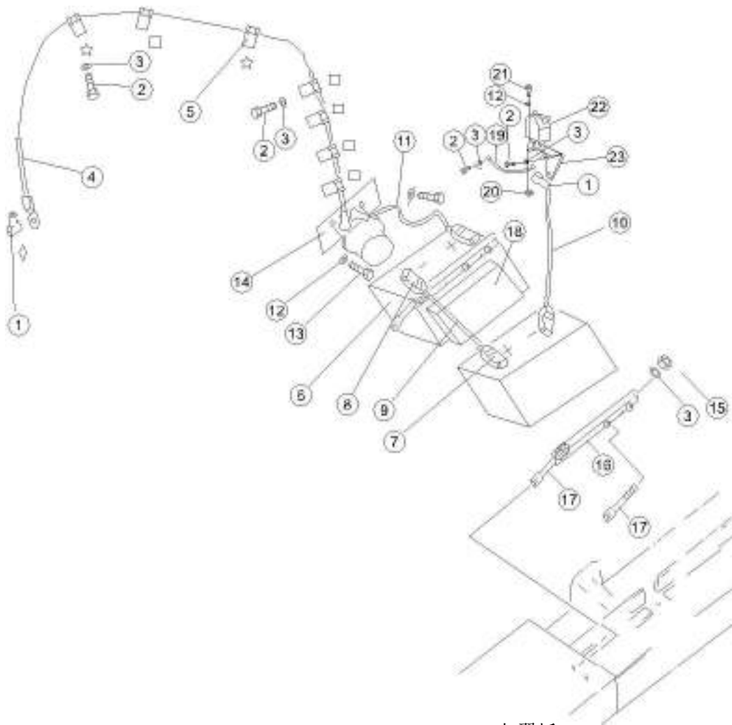
左翼板 Fender L.H.
