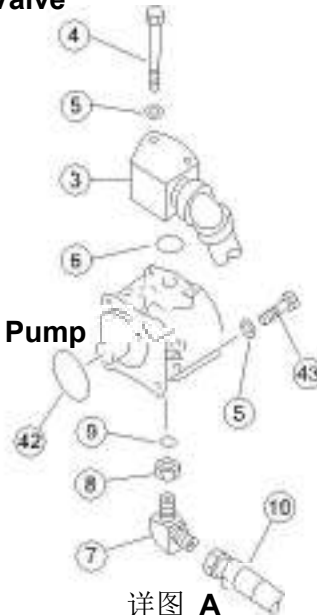
详图 A Detail A
