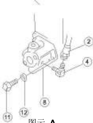
图示 A Detail A
