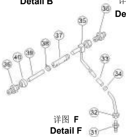
详图 B Detail B
