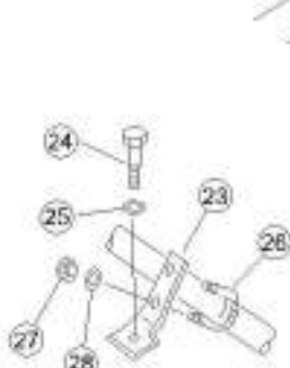
详图 B Detail B
